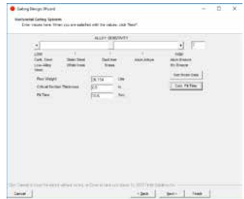
Figura 1. Selección de Aleación y Cálculo de tiempo óptimo de Llenado (OFT)..
